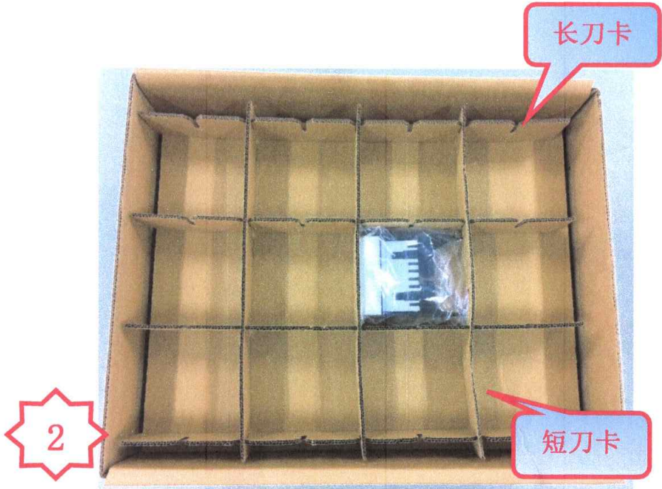
图二, 将 BEZEL 按照每层 12PCS, 每箱 3 层的方式进行包装, 同时在底层和每层的顶部放一块隔板, 共 4 块隔板。
